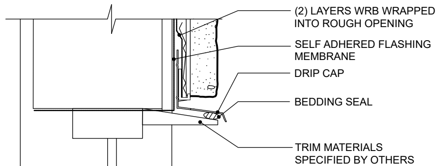
JAMB DETAIL
