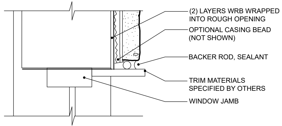
JAMB DETAIL
